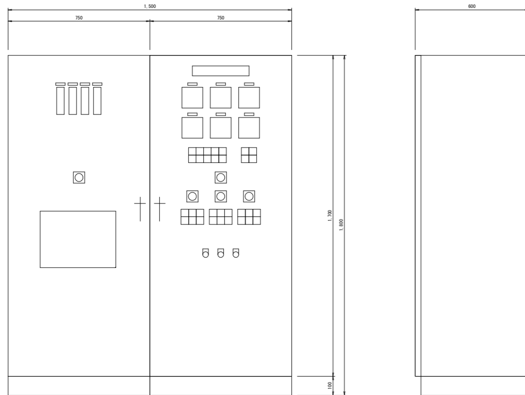
流量調節制御盤
